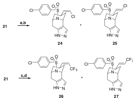
Scheme 6. Reagents and conditions: (a) ClCH 2 PPh 3 Cl, n BuLi, THF, 0 °C, 1 h, 53%; (b) HCl/dioxane, CH 3 OH, 2 h, 60 °C; (c) Ph 2 P(O)CH 2 CF 3 , TBAF, THF, –40 °C, 4 h, 12%; (d) HCl/dioxane, CH 3 OH, 60 °C, 2 h.
